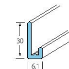
Alu startprofiel 10x3m. Art.nr.: 404
