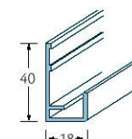
Startprofiel verticaal 5x6m. Art.nr.: 413
